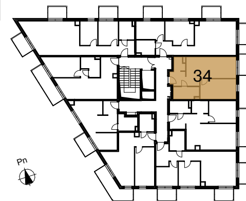
Rzut kondygnacji
