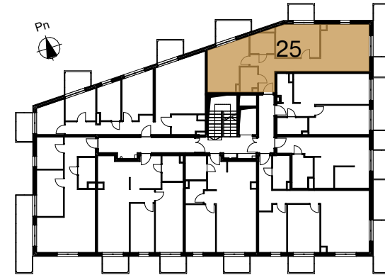
Rzut kondygnacji
