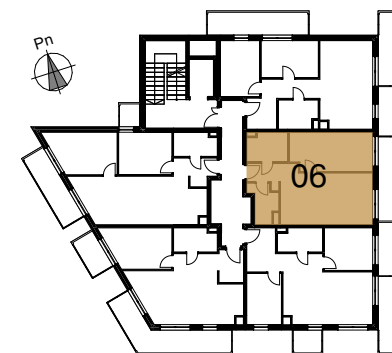
Rzut kondygnacji
