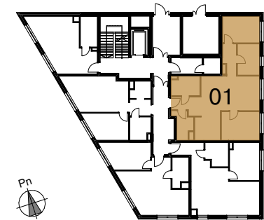
Rzut kondygnacji
