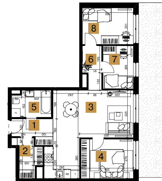
Rzut kondygnacji
