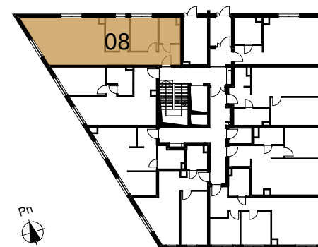
Rzut kondygnacji
