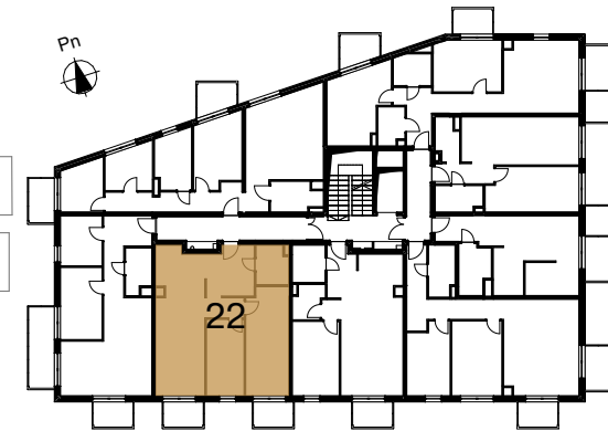
Rzut kondygnacji
