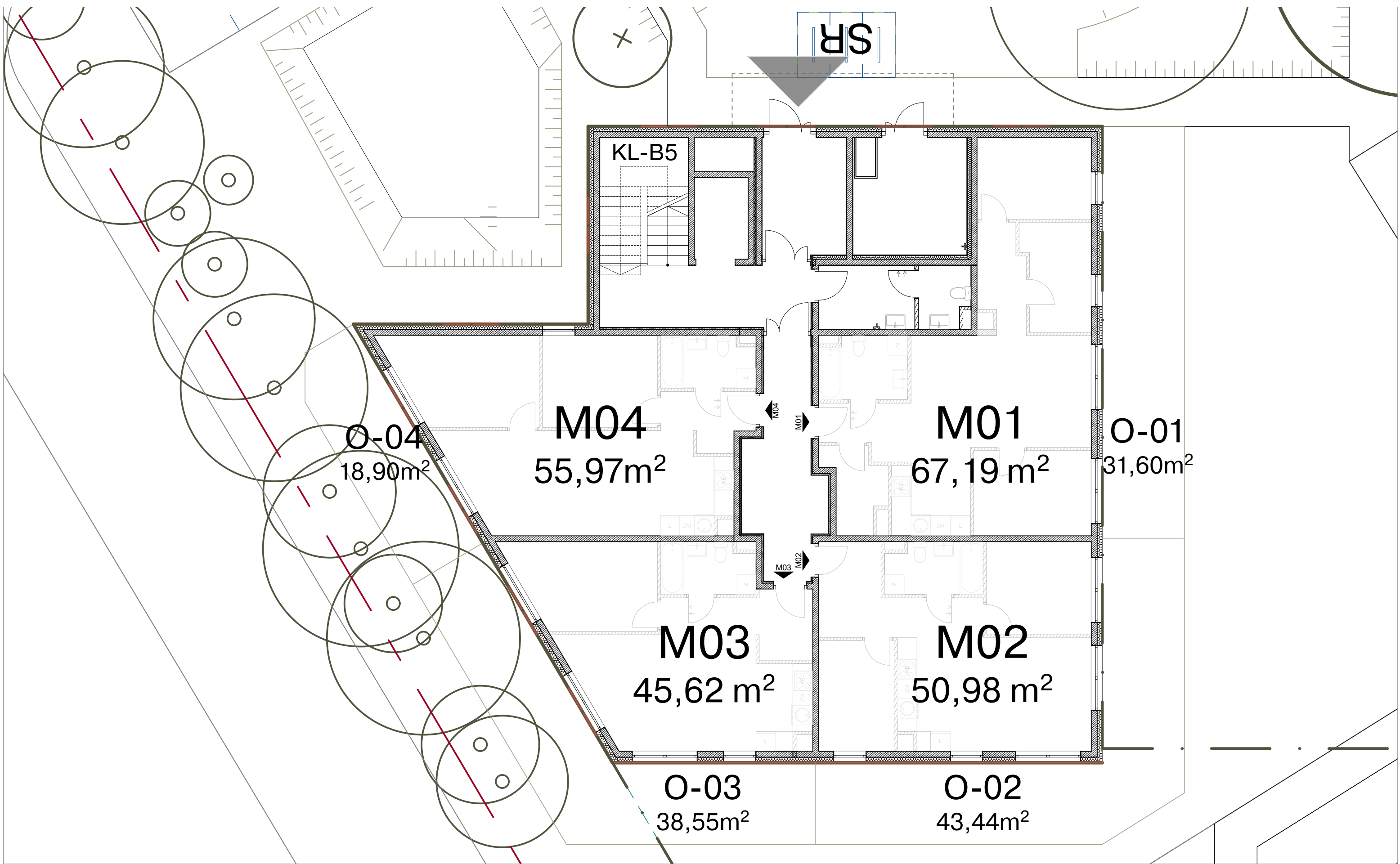
RZUT PARTERU, BUDYNEK B5 - POZIOM 0
