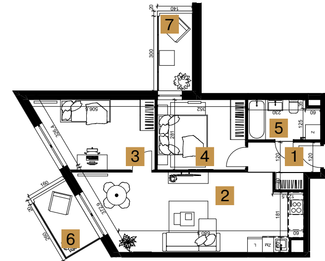
Rzut kondygnacji
