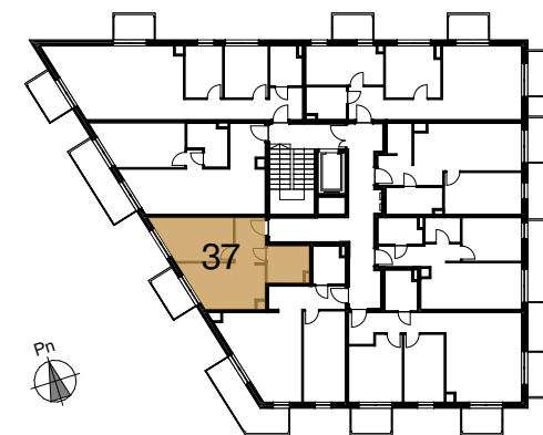
Rzut kondygnacji
